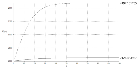
Gambar 4. Plot pertumbuhan populasi pemangsa kedua
