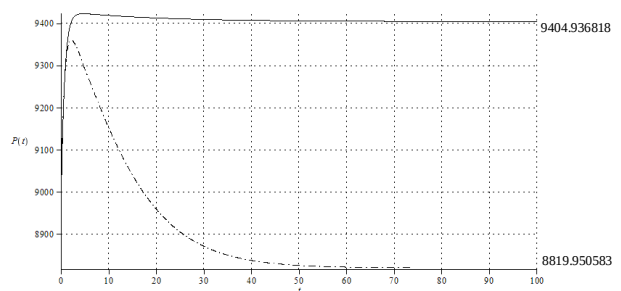
Gambar 2. Plot pertumbuhan populasi mangsa
