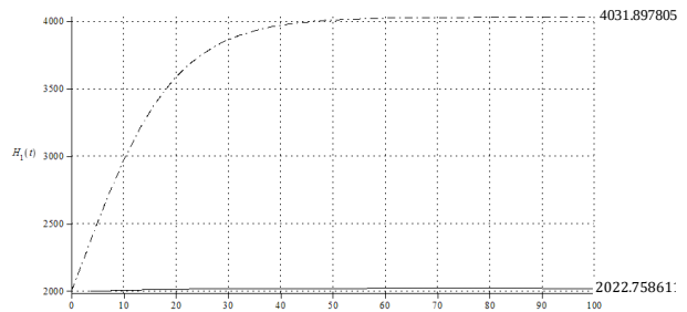
Gambar 3. Plot pertumbuhan populasi pemangsa pertama
